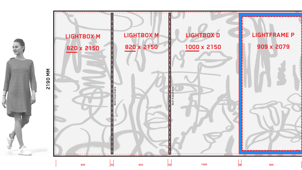
Ansicht und Dateibenennung View and file naming front side MOTIV-LB-820-30-820-30-1000-36-LF-909-4T-3645X2150-1X.PDF
