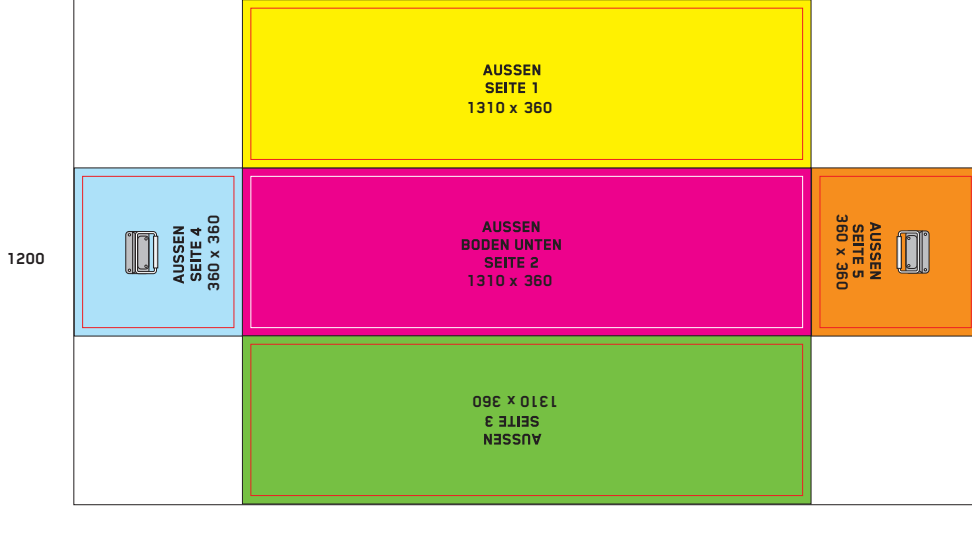
SICHTMASSE ABWICKLUNG CASE ZZGL. 20MM DRUCKERWEITERUNG UMLAUFEND - DATEIGRÖSSE 2150 x 1200 TOTAL SURFACE AREA SIZE SURROUNDING 20MM PRINT EXTENSION - PRINT SIZE 2150 x 1200
