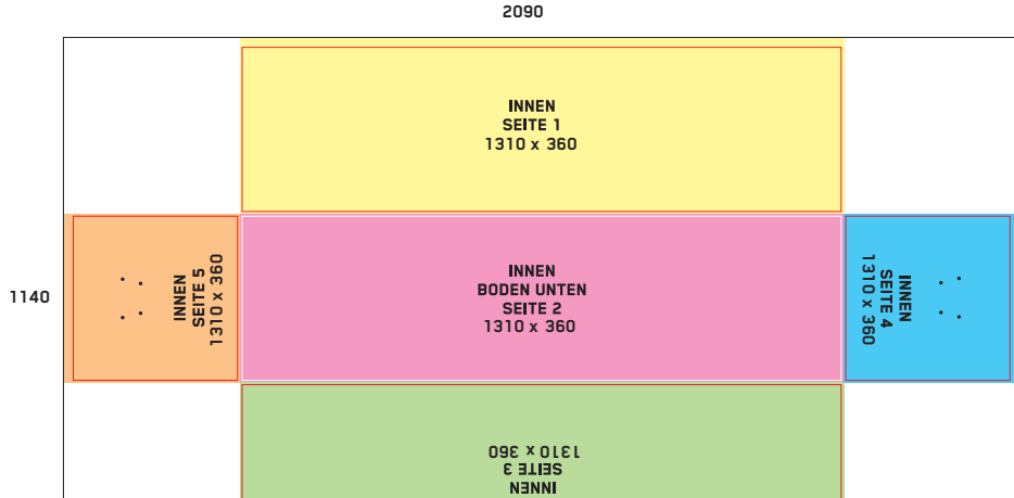
SICHTMASSE ABWICKLUNG CASE ZZGL. 20MM DRUCKERWEITERUNG UMLAUFEND - DATEIGRÖSSE 2090 x 1140 TOTAL SURFACE AREA SIZE SURROUNDING 20MM PRINT EXTENSION - PRINT SIZE 2090 x 1140
