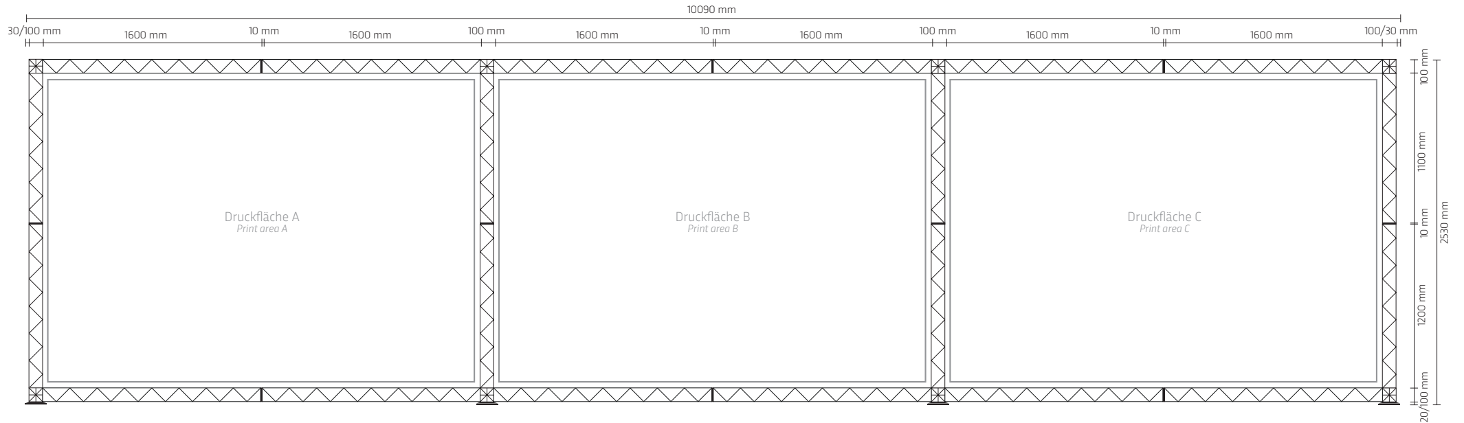
Aufbau Rückwand Assembly rear wall
