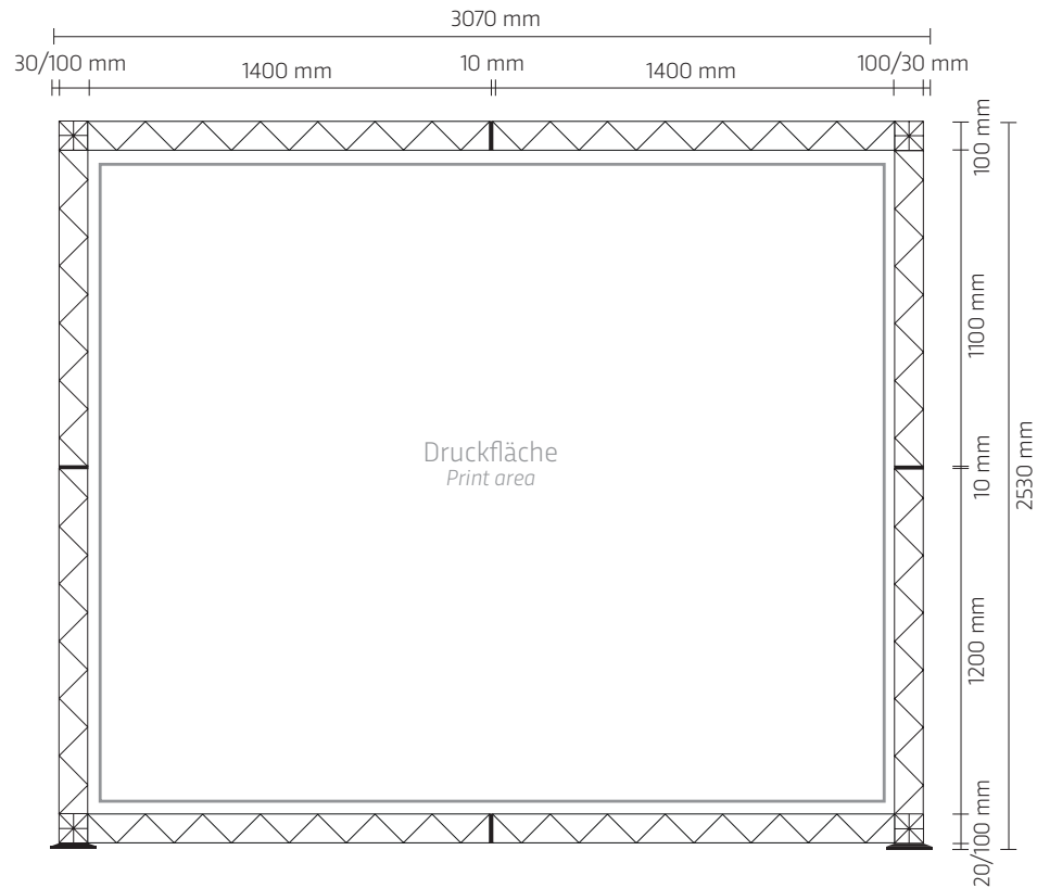
Aufbau Rückwand Assembly rear wall
