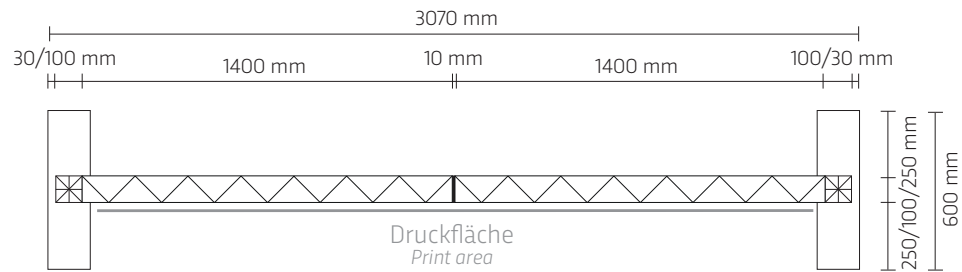
Übersicht Rückwand Overview rear wall
