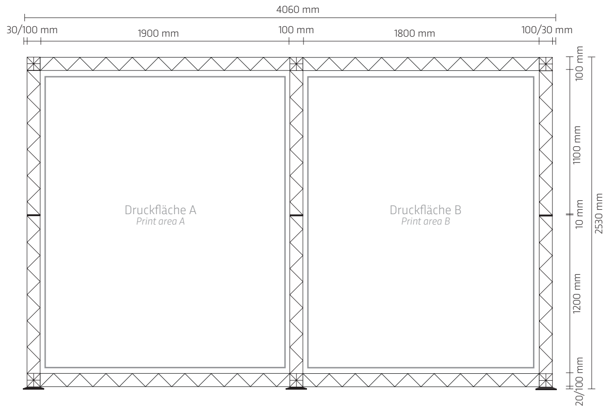
Aufbau Rückwand Assembly rear wall
