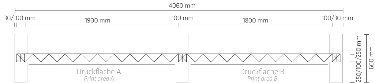
Übersicht Rückwand Overview rear wall
