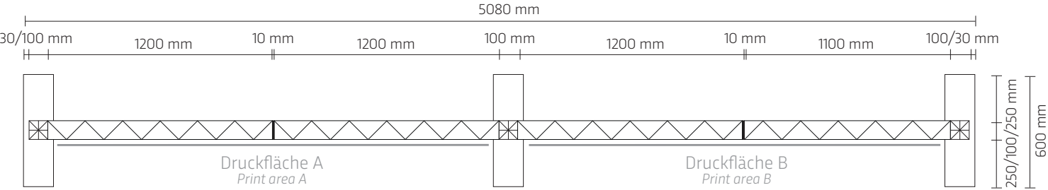
Übersicht Rückwand Overview rear wall
