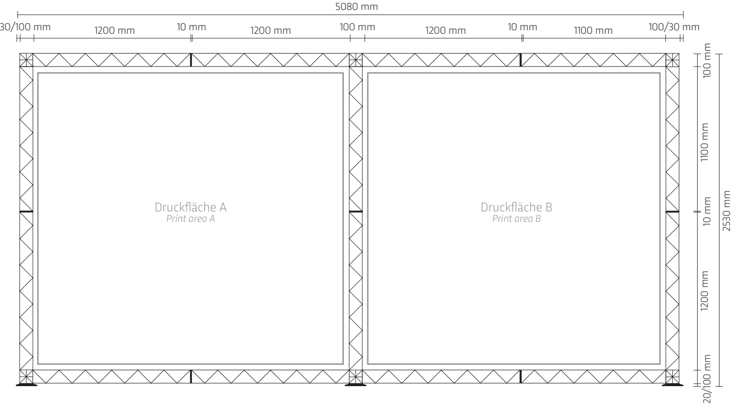
Aufbau Rückwand Assembly rear wall
