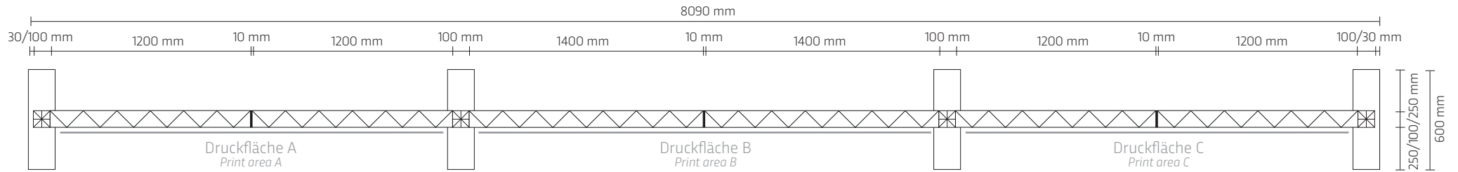
Übersicht Rückwand Overview rear wall
