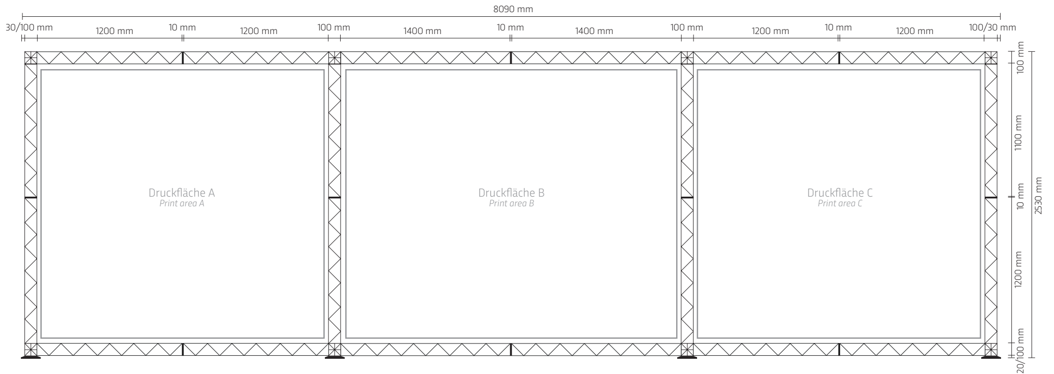
Aufbau Rückwand Assembly rear wall
