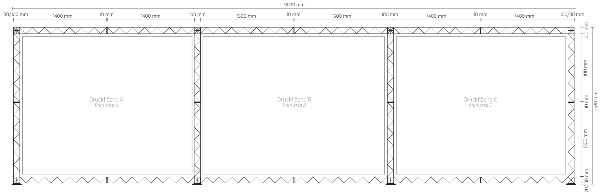
Aufbau Rückwand Assembly rear wall
