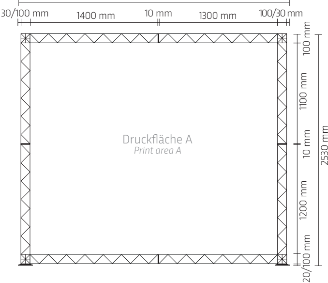
Seitenwand links Side wall left side
