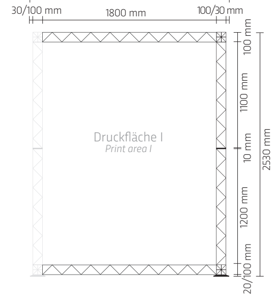
Seitenwand rechts
