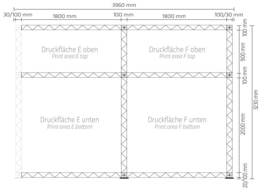
Seitenwand rechts Side wall right side
