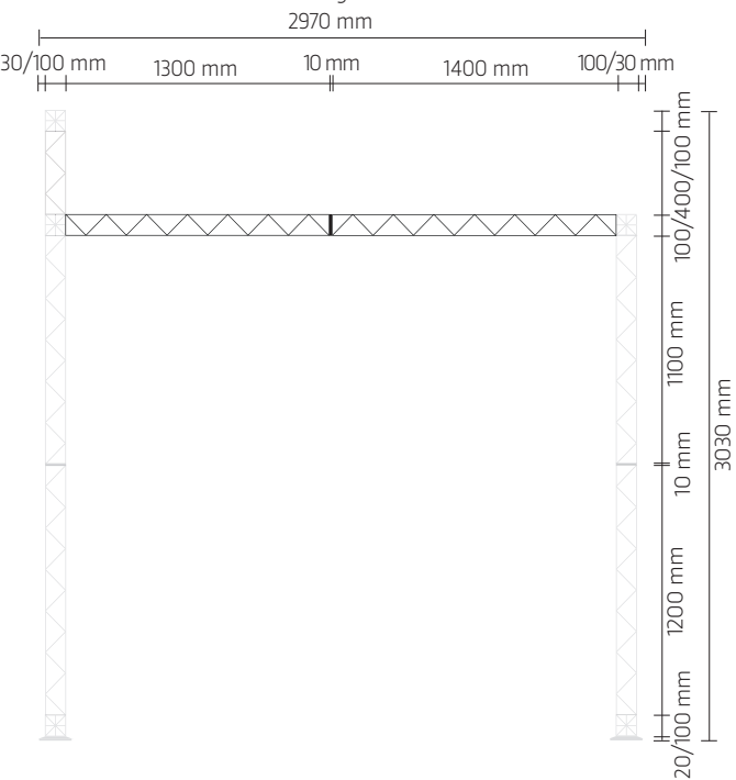
Blende Seite rechts Blende right side
