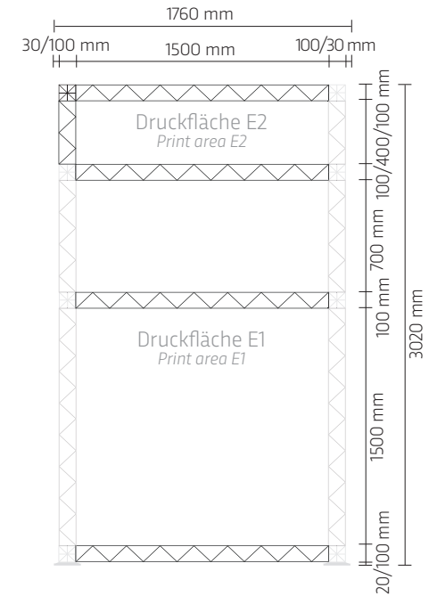
Kabine Vorderseite Cabin front side
