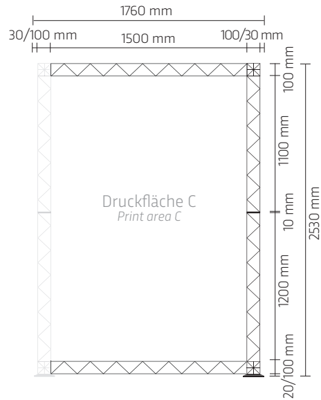
Kabine Rückseite Cabin rear side
