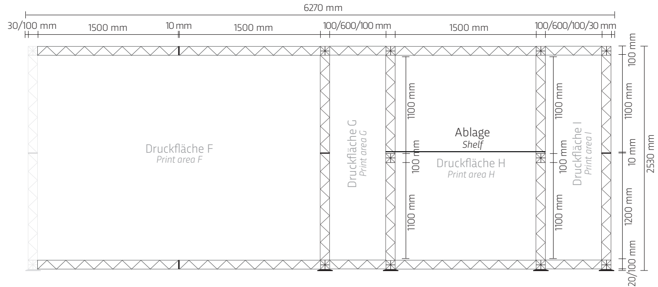
Rückwand Rear wall
