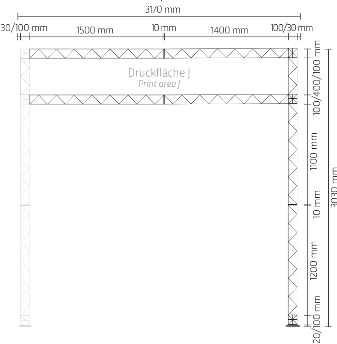
Blende Vorderseite Blende front side
