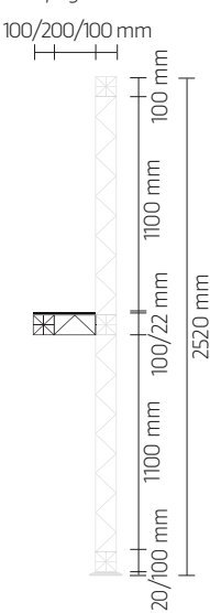
Ablage rechte Seite Shelf right side
