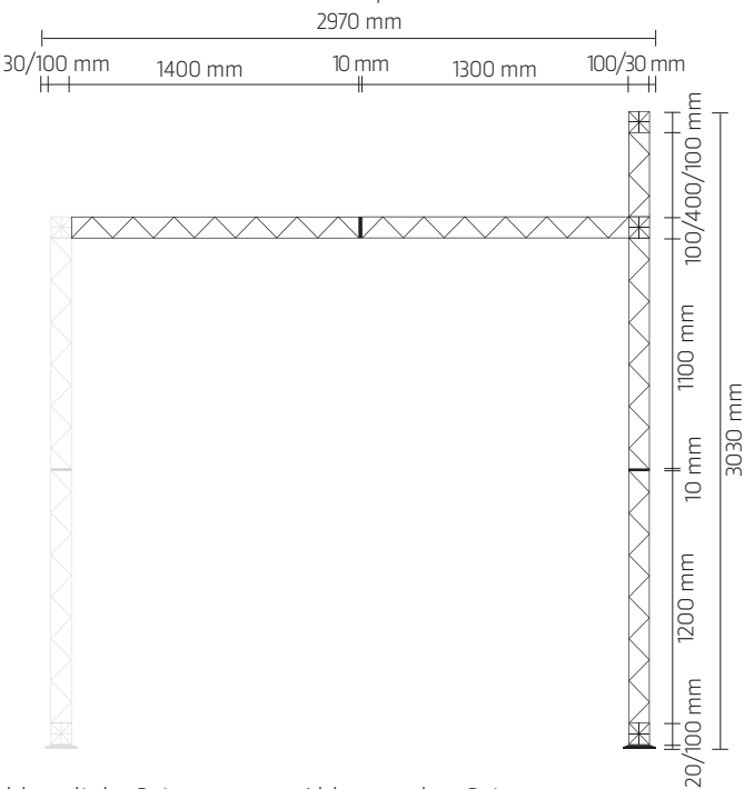
Ablage linke Seite Shelf left side
