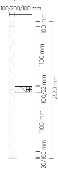
Ablage linke Seite Shelf left side
