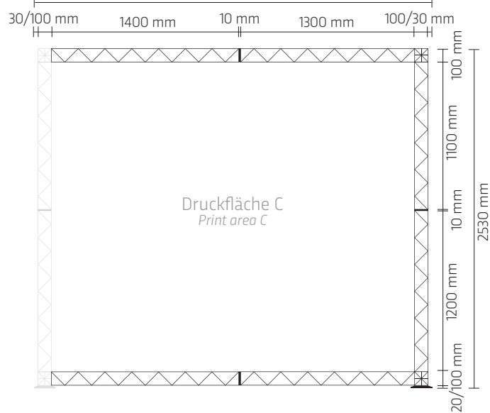
Kabine Rückseite Cabin rear side
