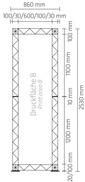
Kabine Seite links Cabin left side
