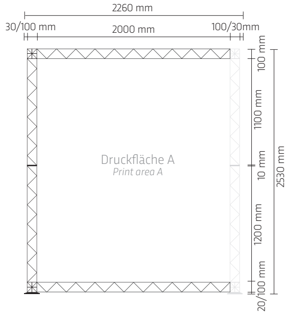
Kabine Seite links Cabin left side
