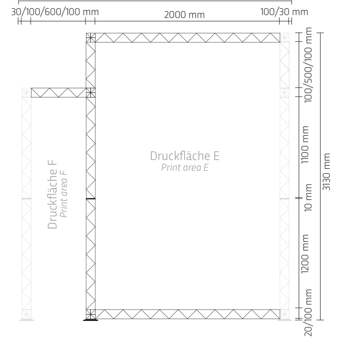
Kabine Vorderseite Cabin front side
