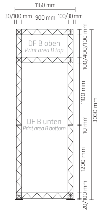
Kabine Seite links Cabin left side
