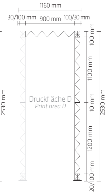
Kabine Seite rechts Cabin right side
