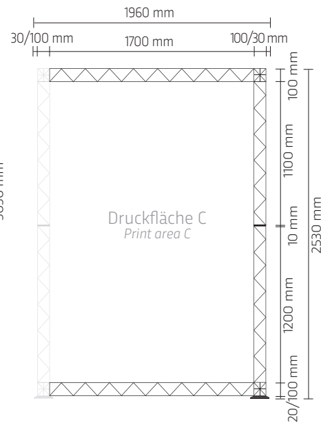
Kabine Rückseite Cabin rear side
