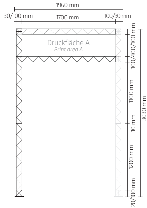
Seitenwand links Side wall left side
