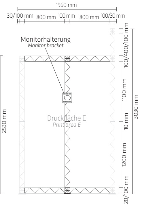
Kabine Vorderseite Cabin front side
