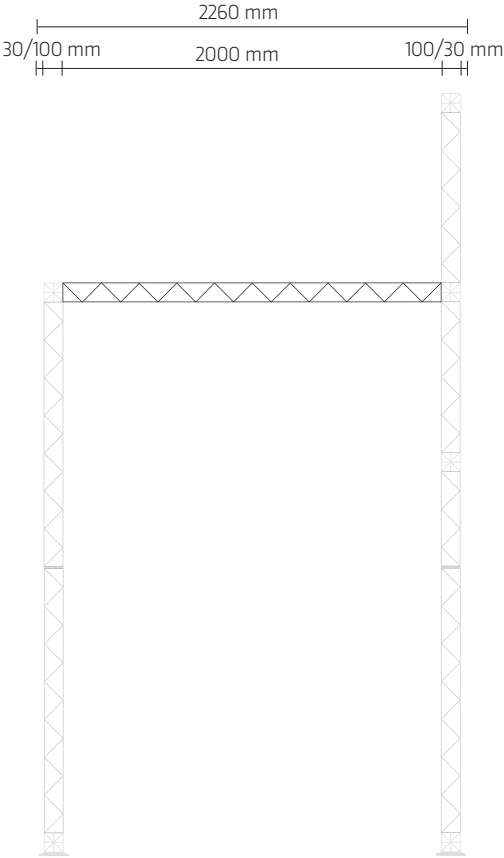
Verbindungselement 1 Connection element 1
