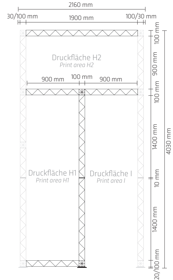
Kabine Rückseite Cabin rear side
