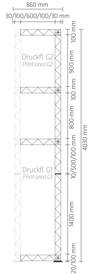
Kabine Seite links Cabin left side
