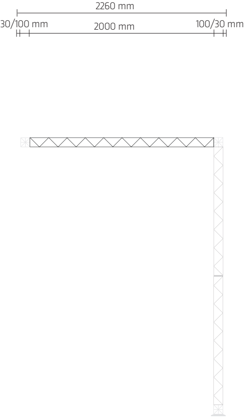
Verbindungselement 2 Connection element 2
