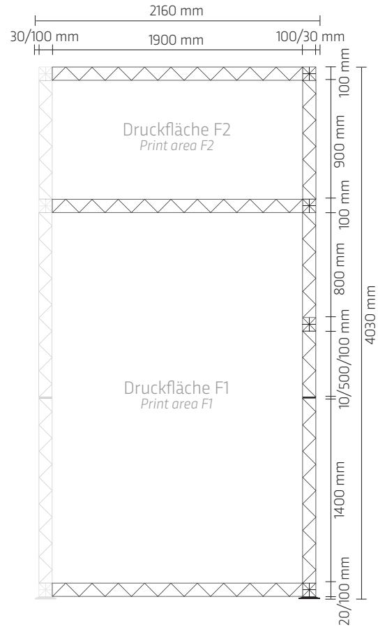
Kabine Vorderseite Cabin front side
