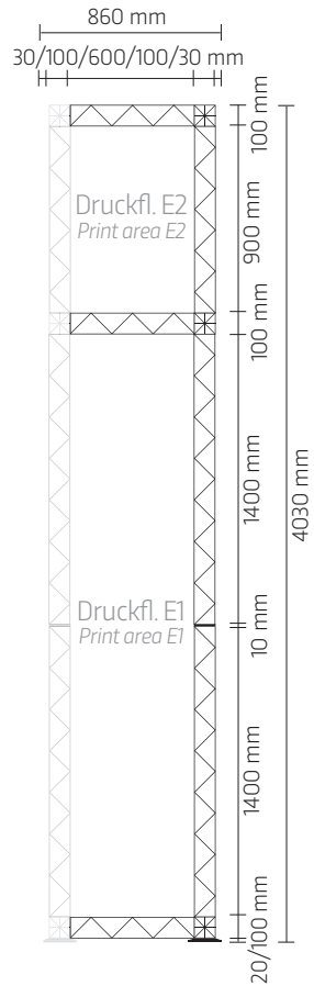
Kabine Seite rechts Cabin right side
