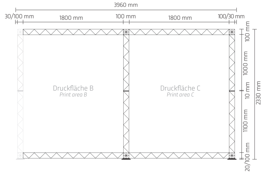
Rückwand Rear wall
