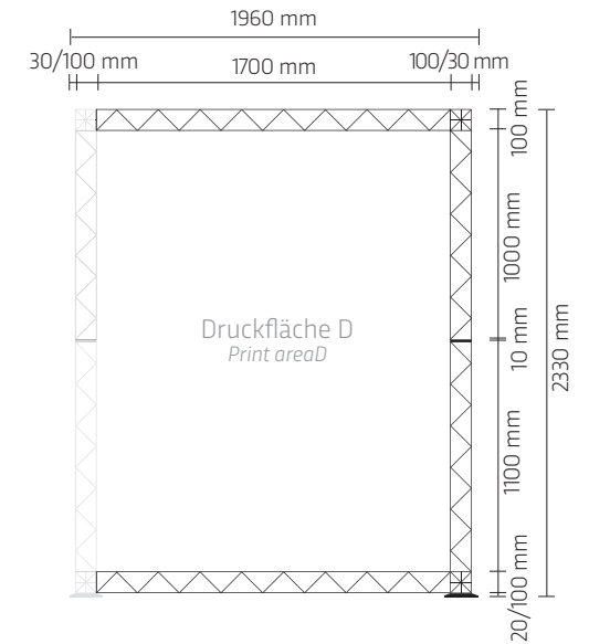
Seitenwand rechts Side wall right side
