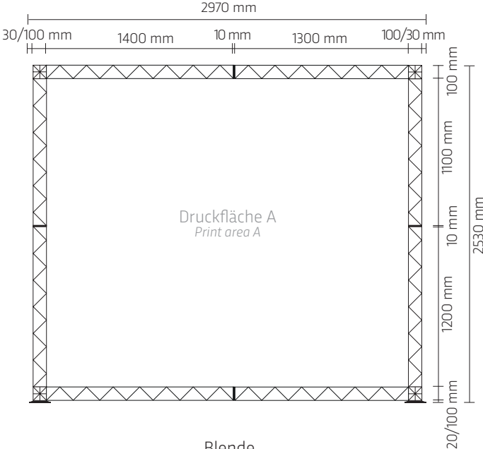
Blende Blende
