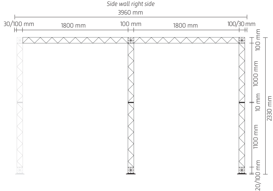
Seitenwand rechts Side wall right side
