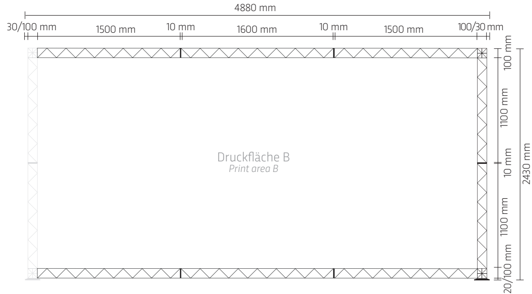
Turm Seite links Tower left side
