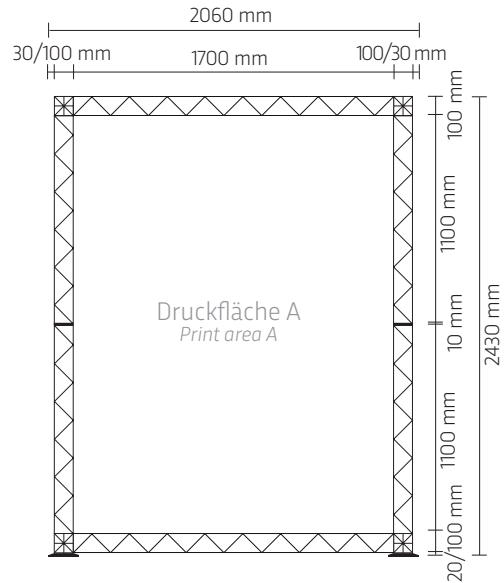
Turm Vorderseite Tower front side
