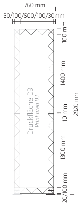
Turm Rückseite Tower rear side
