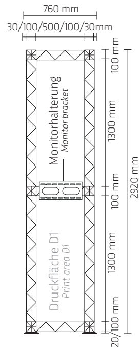
Turm Vorderseite Tower front side
