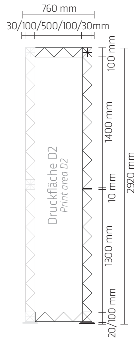
Turm Seite rechts Tower right side
