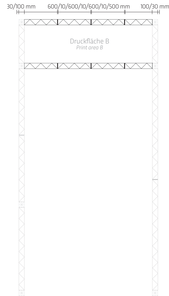
Verbindung Turm 1 zu Turm 2 Connection tower 1 to tower 2
