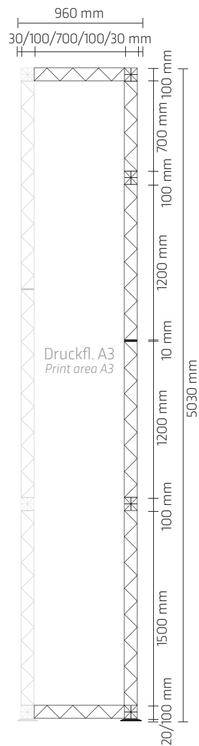
Turm 1 Seite rechts Tower 1 right side
