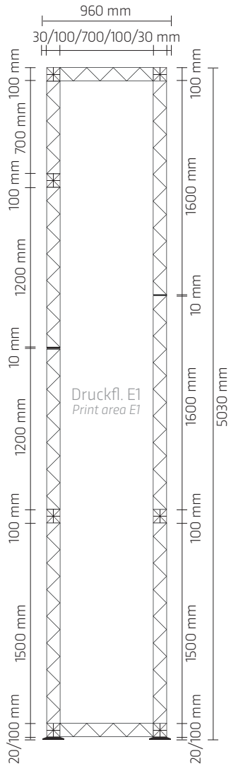
Turm 3 Seite links Tower 3 left side
