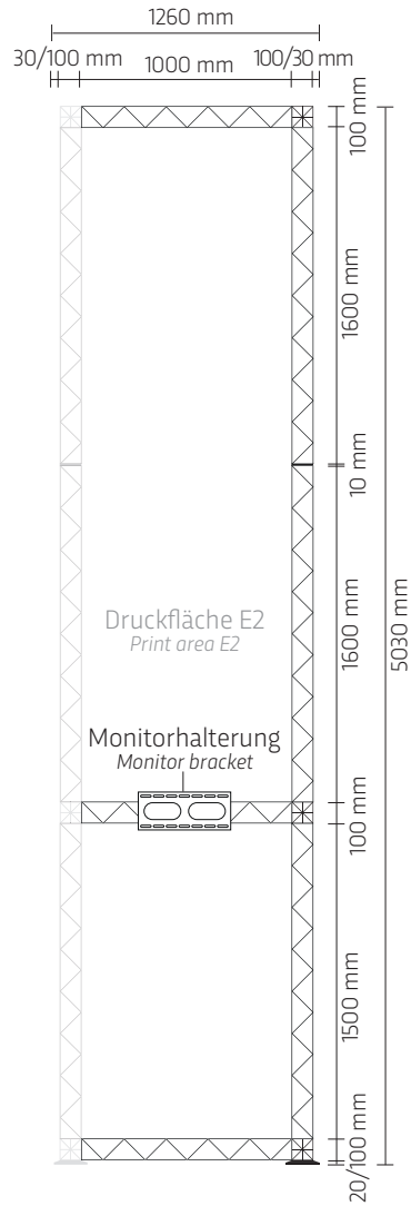
Turm 3 Rückseite Tower 3 rear side
