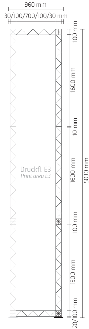
Turm 3 Seite rechts Tower 3 right side
