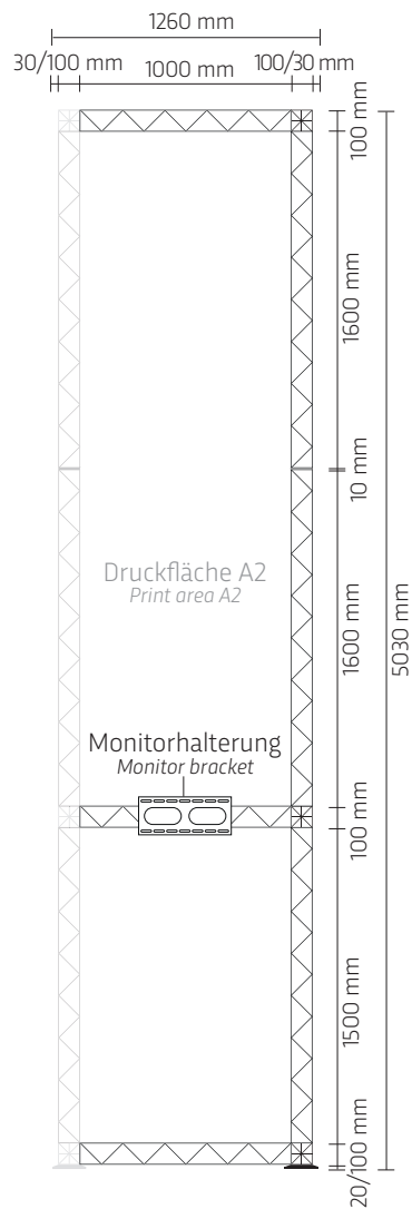
Turm 1 Rückseite Tower 1 rear side
