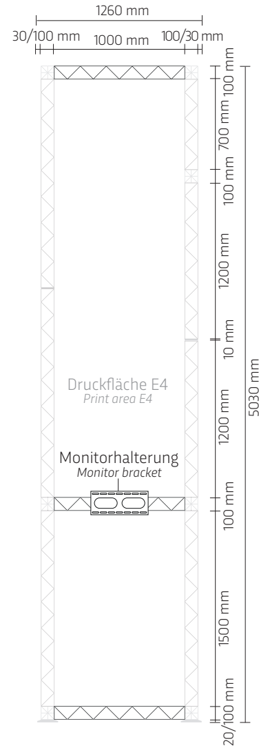
Turm 3 Vorderseite Tower 3 front side
