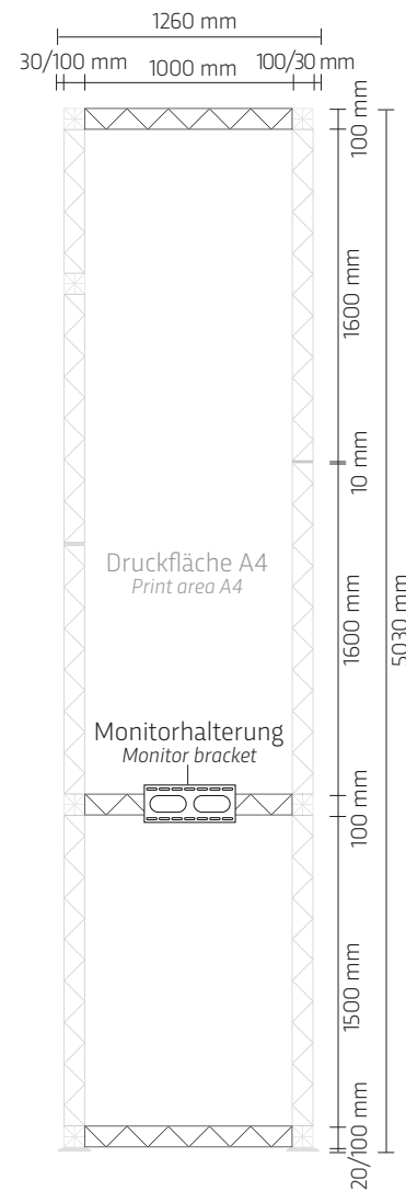
Turm 1 Vorderseite Tower 1 front side
