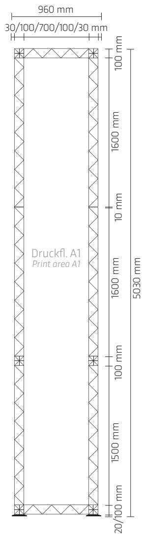
Turm 1 Seite links Tower 1 left side
