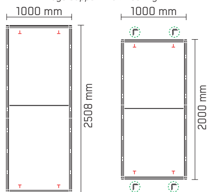
Brücke Stützwand / Decke Bridge support wall / ceiling
