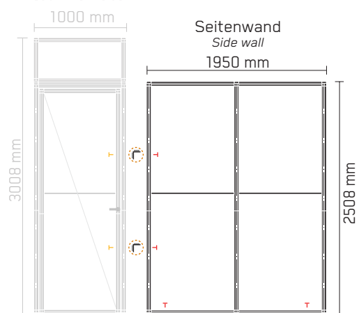
Kabine Vorderseite Cabin front side
