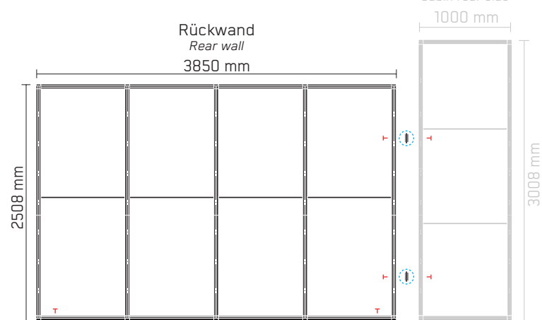
Kabine Rückseite Cabin rear side
