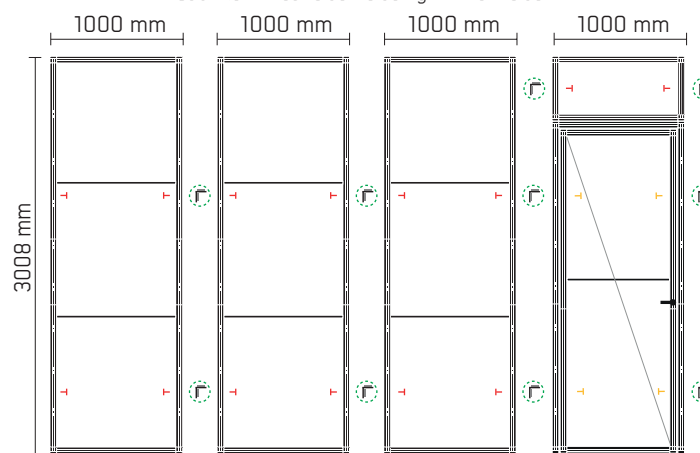
Kabine Seite links / Rückseite / Seite rechts / Vorderseite Cabin left / rear side / side right / front side
