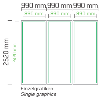
Kabine Seiten + Rückseite Cabin sides + rear side
