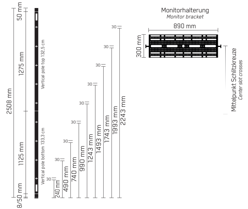
Seitenansicht Profil Side view profile
