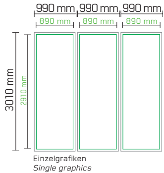
Kabine Seiten + Rückseite Cabin sides + rear side
