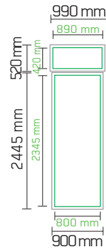
Kabine Türblatt / Aufsatz Cabin door leaf / attachment
